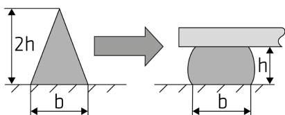
Abbildung 1: Empfohlener Klebstoffauftrag
